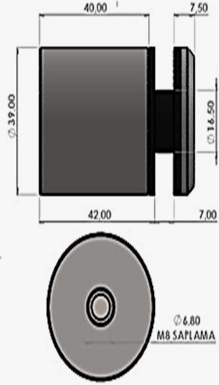
GENEL ÖLÇÜLER
